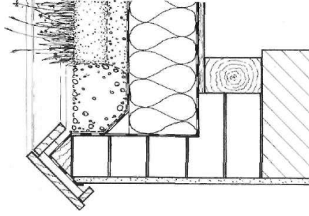
6.8 Detalle de pretli
