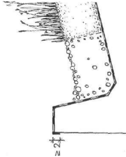
6.2 Conformación de la membrana de techo contra el canalón
