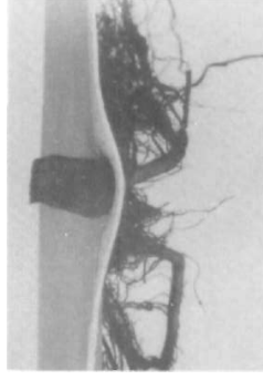
4.6 Perforación en una unión pegada de dos láminas de PVC producida por una raíz (Pennigsfeld et al. 1981)
