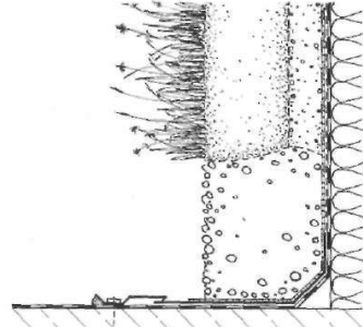
6.3, 6.4 Encuentros de borde con muros que continúan
