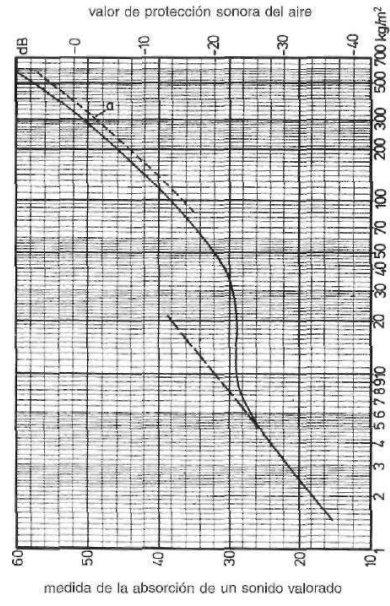
2.6 Dependencia de la absorción acústica del aire con el peso de las superficies (Gosele, Schüle 1983)
