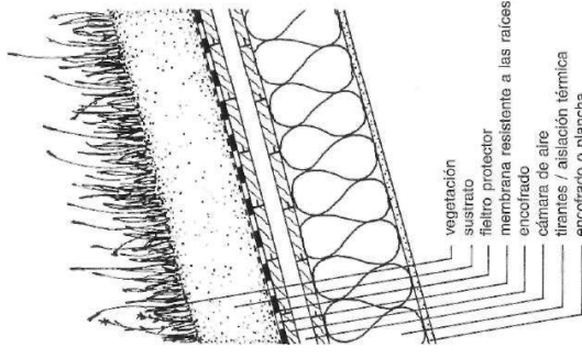
4.3 Típica formación de un techo frío con enjardinado
